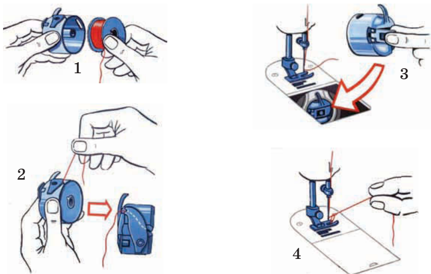
Рис. 64. Заправка нижней нитки
