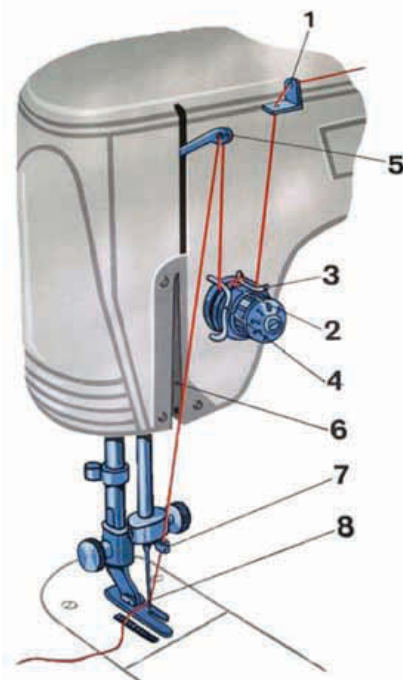
Рис. 63. Заправка верхней нитки
