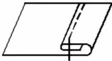
Рис. 71. Шов вподгибку с закрытым срезом
