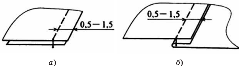
Рис. 70 а, б. Стачной шов в заутюжку
