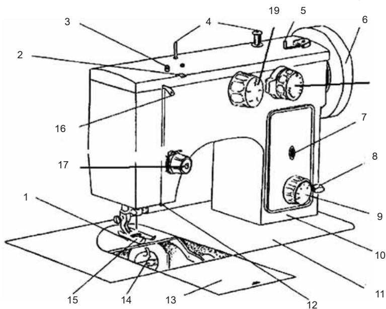
Рис. 62. Основные узлы швейной машины
